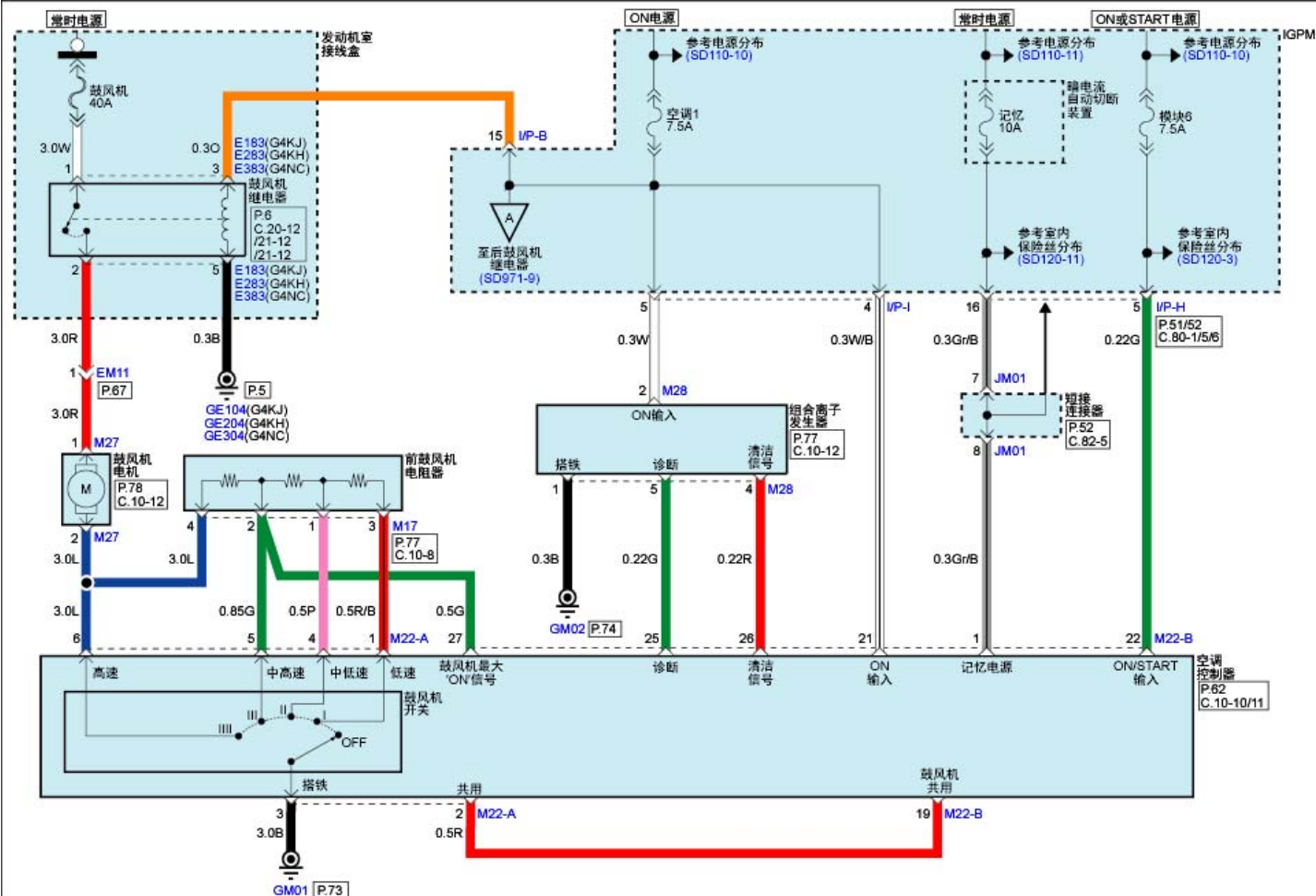
空调控制系统(手动)(1)
